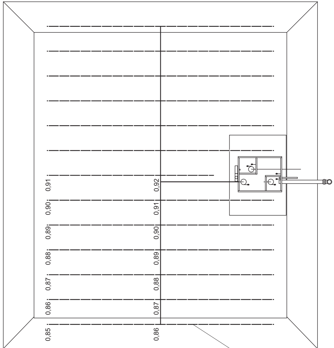
Zulaufverteilung mit Bohrungen \varnothing 5 mm
