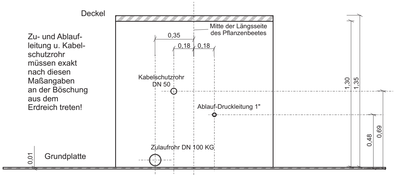
Schachtmodul
