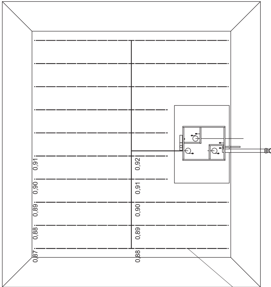
Zulaufverteilung mit Bohrungen \varnothing 5 mm
