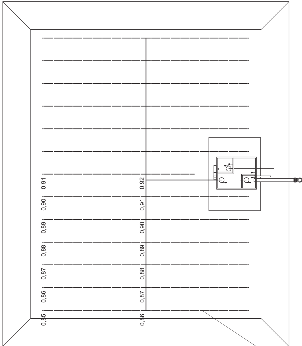
Zulaufverteilung mit Bohrungen \varnothing 5 mm
